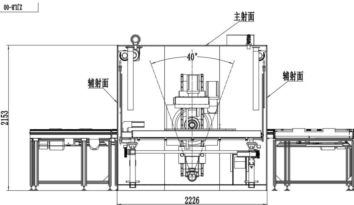
图 10-2 铅房剖面图
