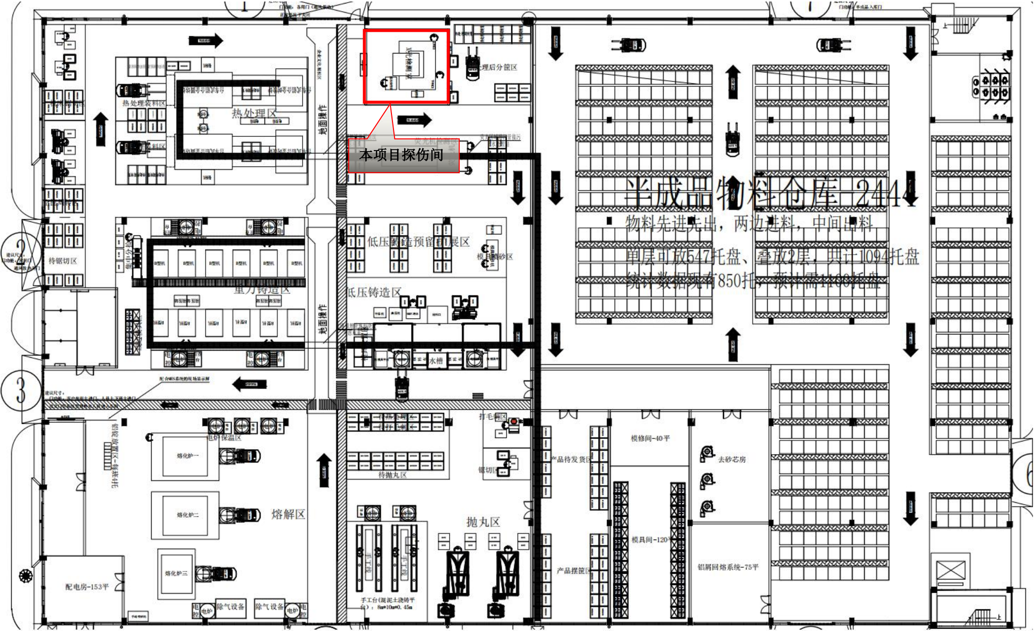
附图 4：铸造车间平面布置图
