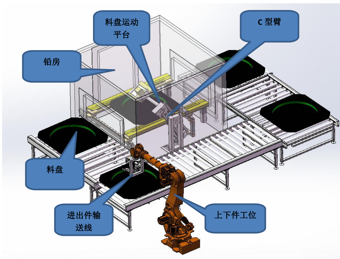
图 9-1 本项目探伤设备示意图
