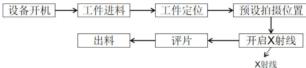
图 9-4 探伤工艺流程简图
