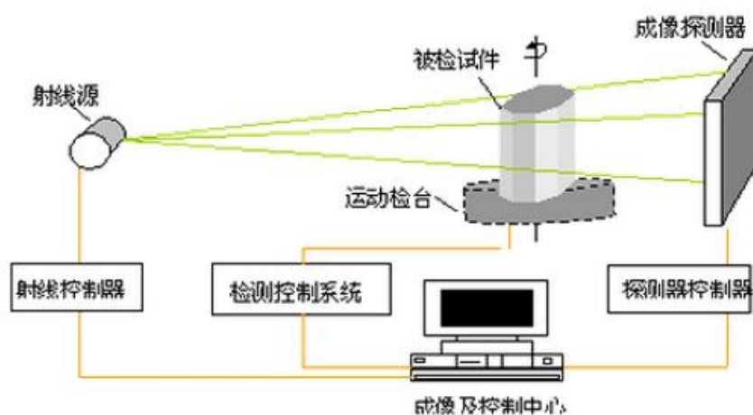
图 9-3 本项目探伤设备工作原理
