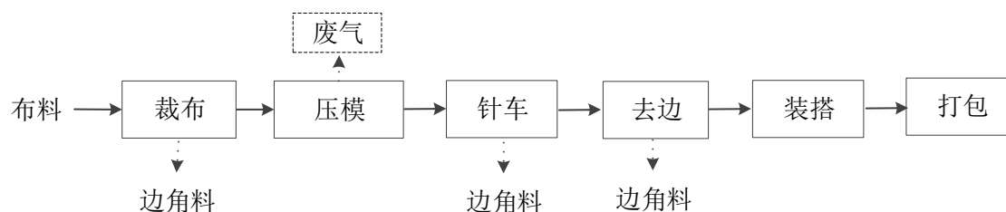
图 2.2.1-3 布箱包工艺流程图
