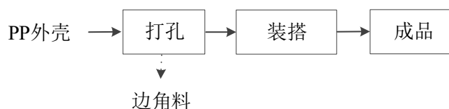
图 2.2.1-3 PP 箱包工艺流程图
