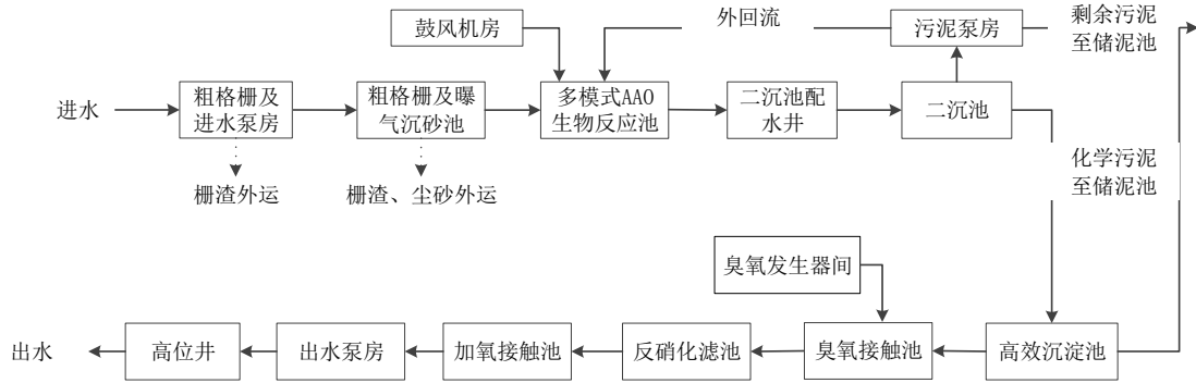
图 4.2.2-1 污水处理工艺流程图
