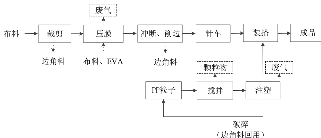
图 1 布箱包工艺流程图
