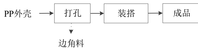
图 3 PP 箱包工艺流程图
