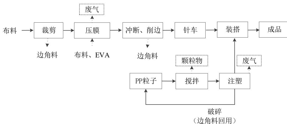
图 2.2.1-1 布箱包工艺流程图
