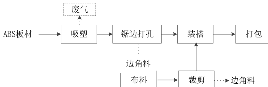
图 2 ABS 拉链箱包工艺流程图
