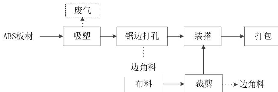
图 2.2.1-2 ABS 拉链箱包工艺流程图
