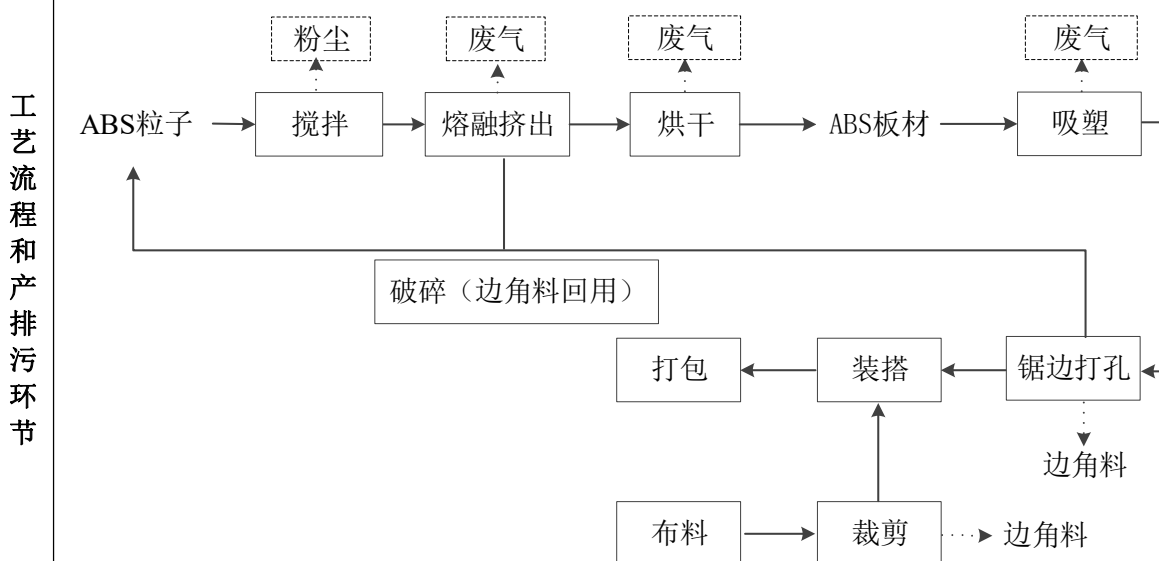
图 2.2.1-1 ABS 拉链箱包工艺流程图
