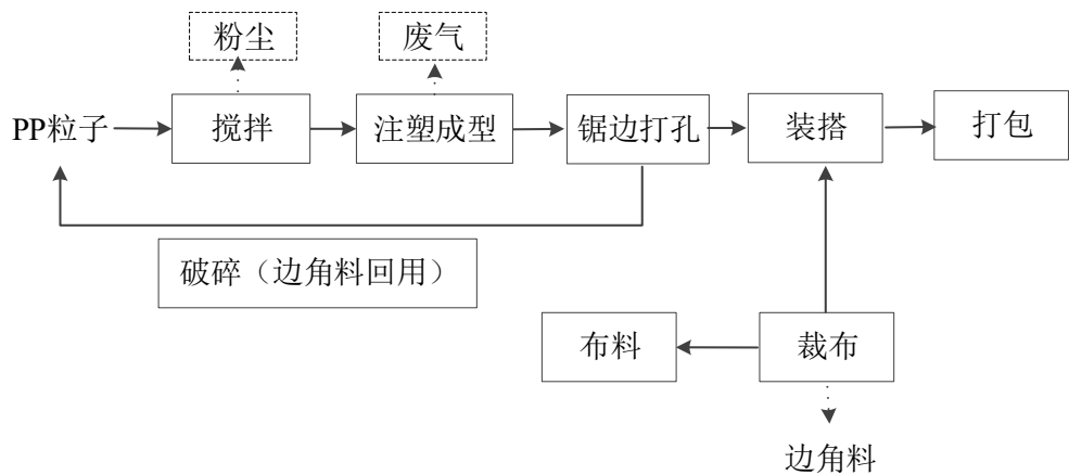
图 2 PP 箱包工艺流程图
