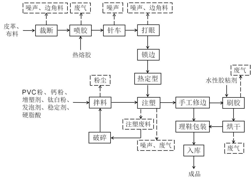
图 1 生产工艺流程图
