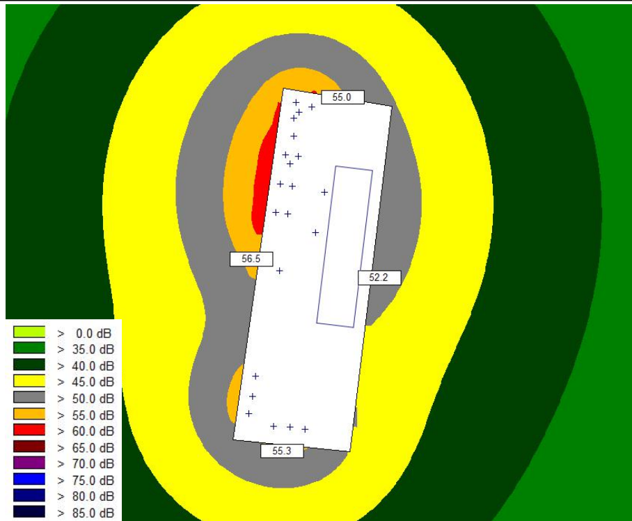
图 4-1 噪声预测结果示意图
