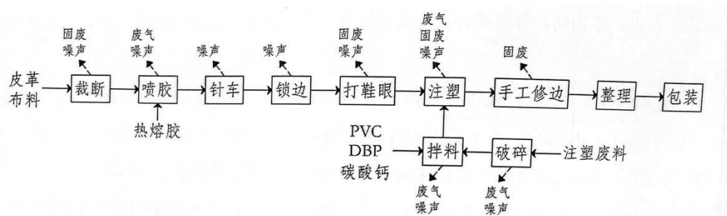
图 2-3 生产工艺流程及产污环节示意图
