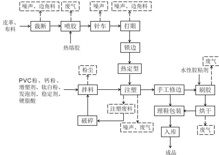
2-2 项目生产工艺流程及产污环节示意图
