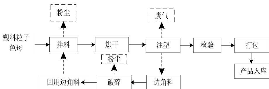
图 2-2 项目迁建前工艺流程图
