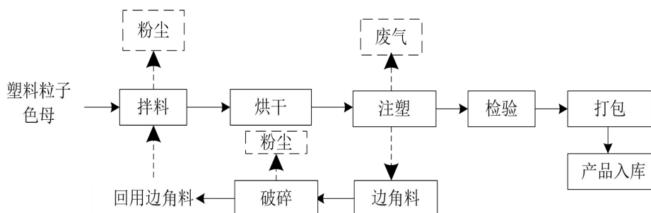
图 2-2 生产工艺流程图
