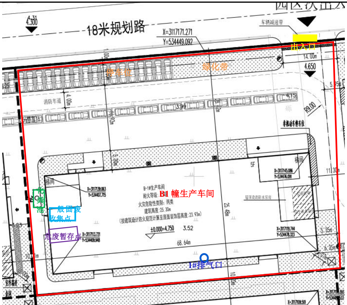
图 2-1 总平面布置图
