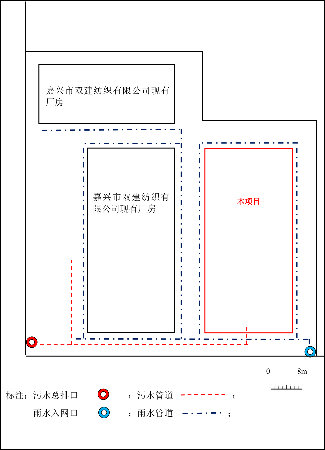
附图 6 雨污水管网图
