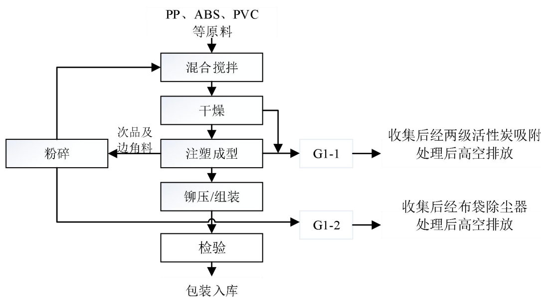
图 2-1 生产工艺流程图
