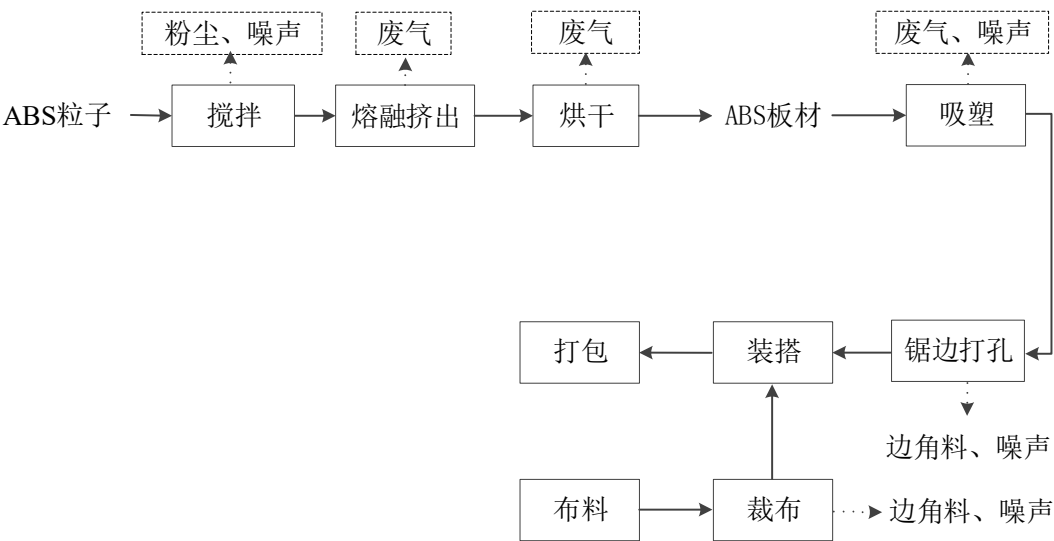
图 2.2.1-1 ABS 拉链箱包工艺流程图
