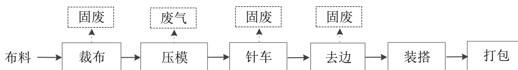
图 2.3.2-2 布箱包工艺流程图
