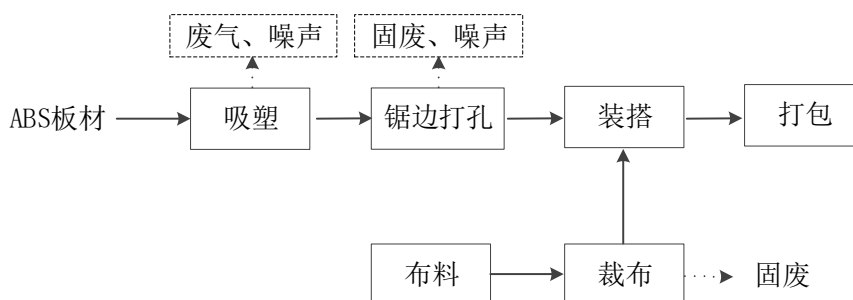
图 2.3.2-1 ABS 拉链箱包工艺流程图
