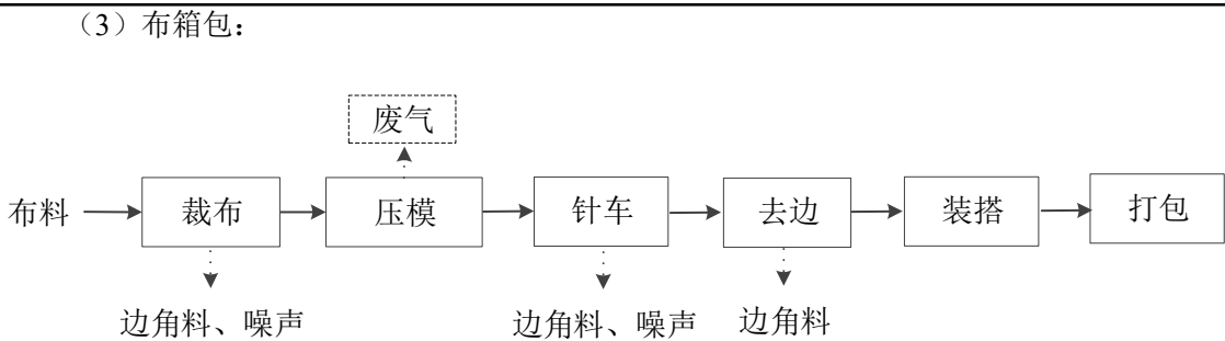
图 2.2.1-3 布箱包工艺流程图
