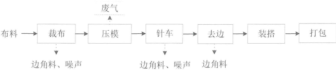
图 3 布箱包工艺流程图
