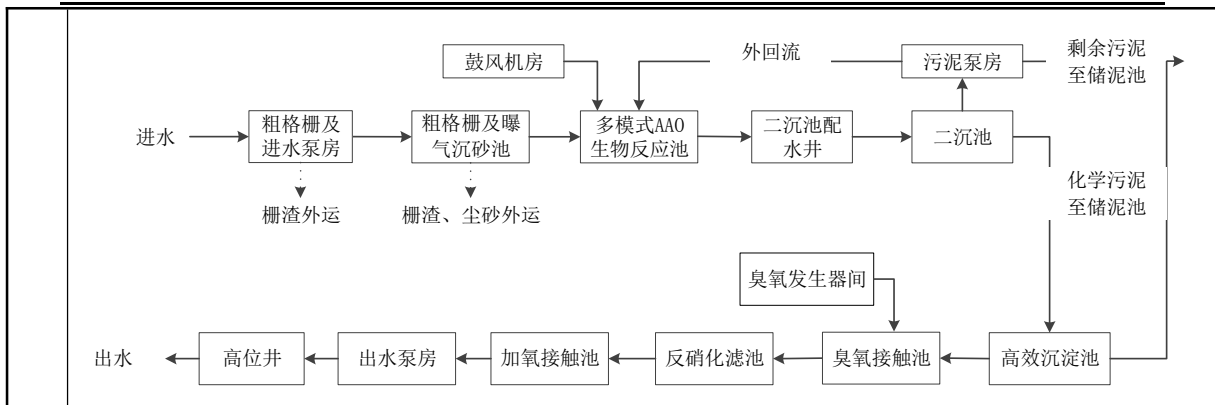
图 4.2.2-1 污水处理工艺流程图
