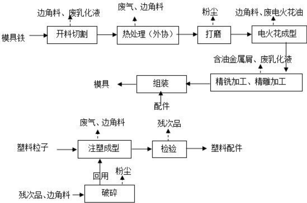
图 2-2 项目迁建前工艺流程图
