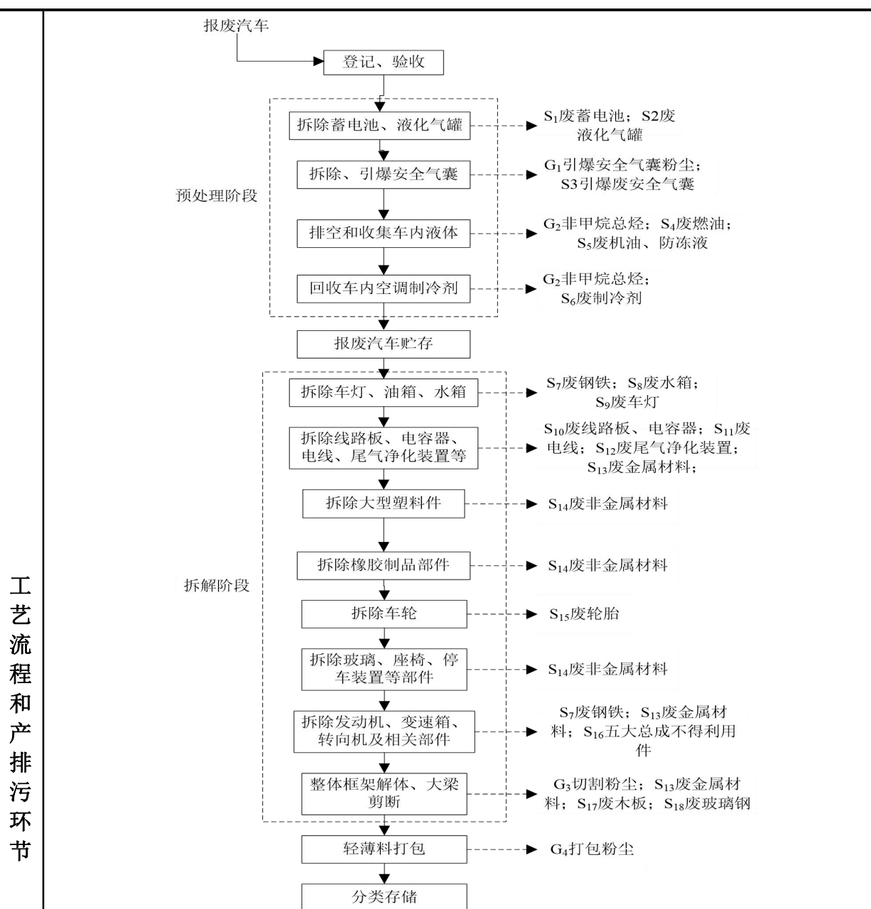
图 2-3 其他燃料报废机动车的处理工艺流程及产污节点示意图
