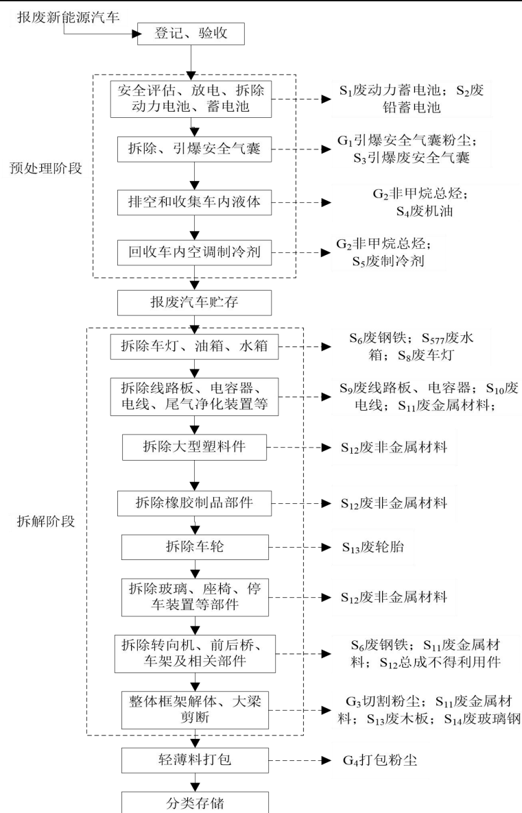
图 2-2 新能源车（电动汽车）的处理工艺流程及产污节点示意图
