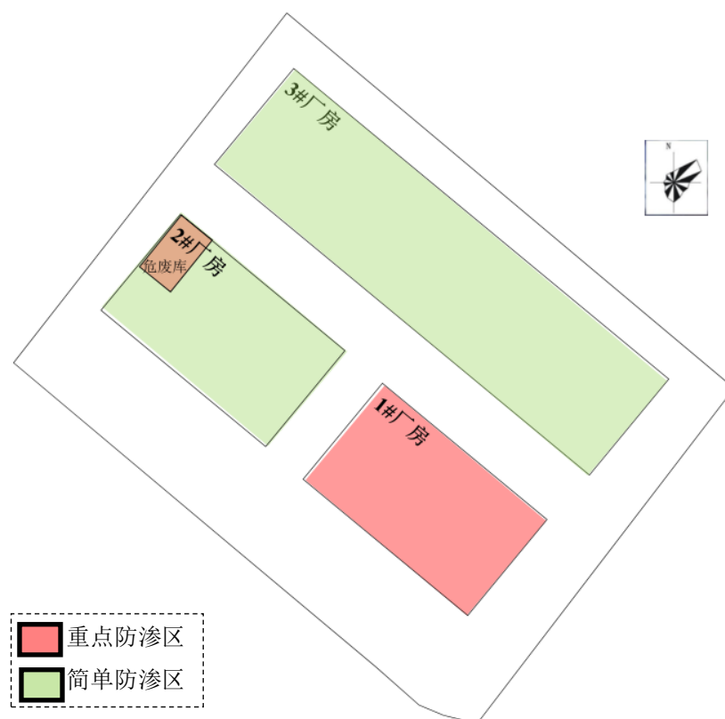
图 4-2 厂区地面地下水、土壤污染防治分区图
