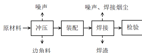
图 2-4 工艺流程图
