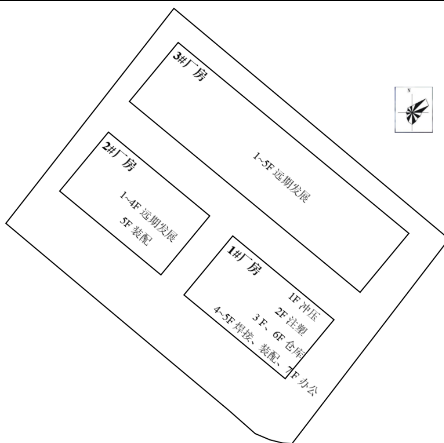
图 2-3 车间布置图
