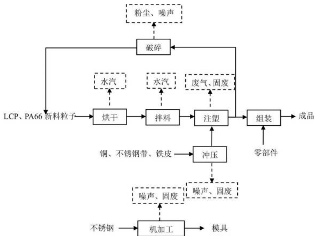
图 2-3 现有工程工艺流程图
