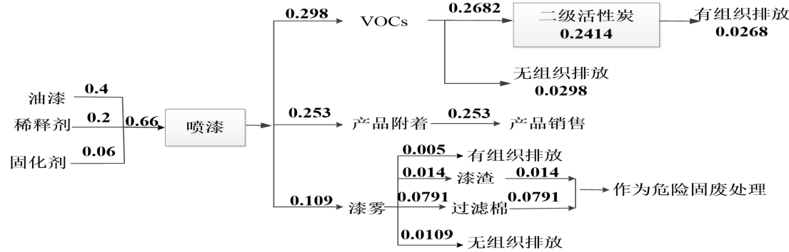
图 2-2 油性漆平衡图（单位：t/a）
