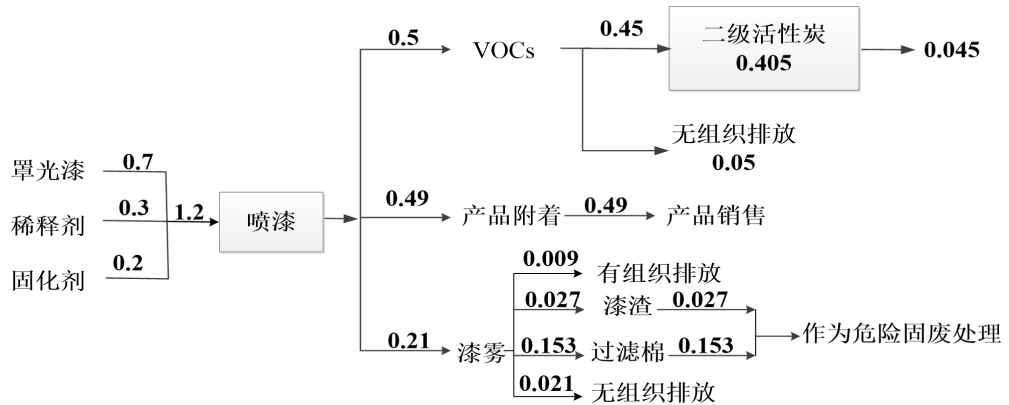
图 2-3 罩光漆平衡图 (单位: t/a)
