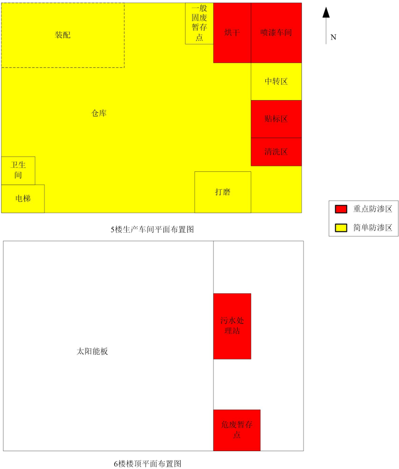
图 4-1 项目厂区地下水污染防渗分区图
