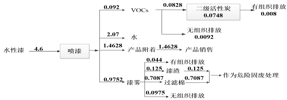
图 2-1 水性漆平衡图（单位：t/a）
