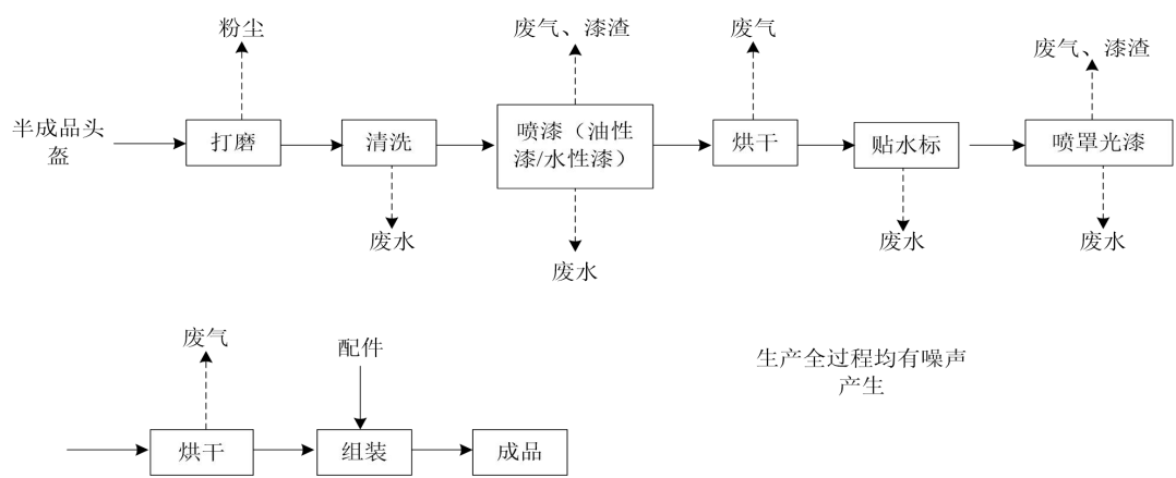
图 2-6 生产工艺流程图
