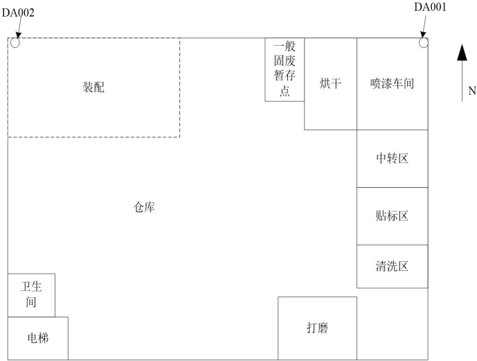
5楼生产车间平面布置图
