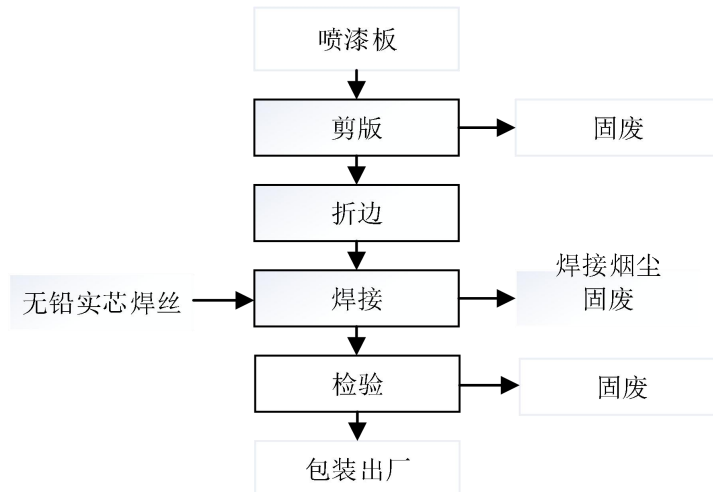
图 2-3 灭火器箱生产工艺流程图
