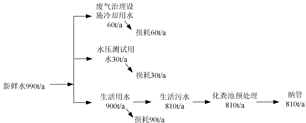
图 2-4 本项目水平衡图
