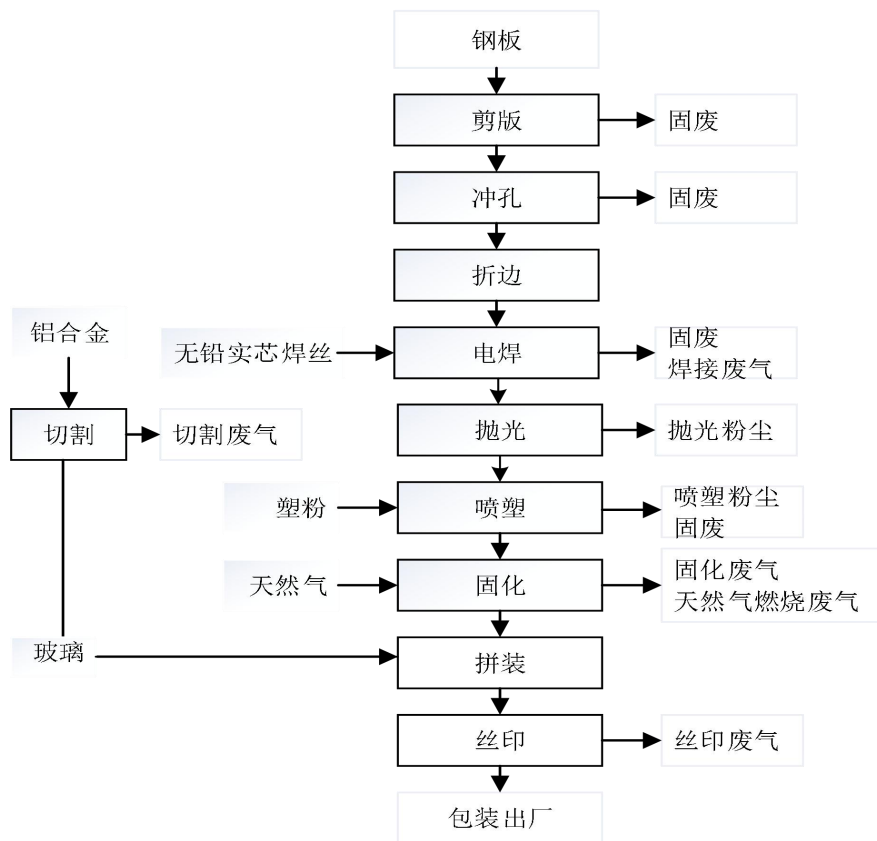
图 2-2 消防箱生产工艺流程图
