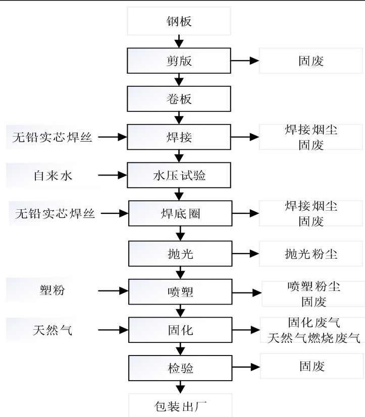
图 2-1 灭火器筒体生产工艺流程图
