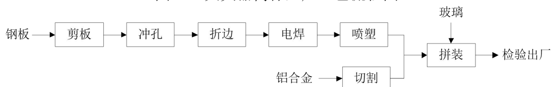
图 2-6 消防箱生产工艺流程图
