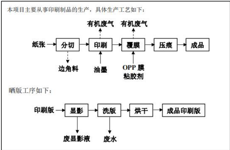
图 2-2 现有项目生产工艺流程图
