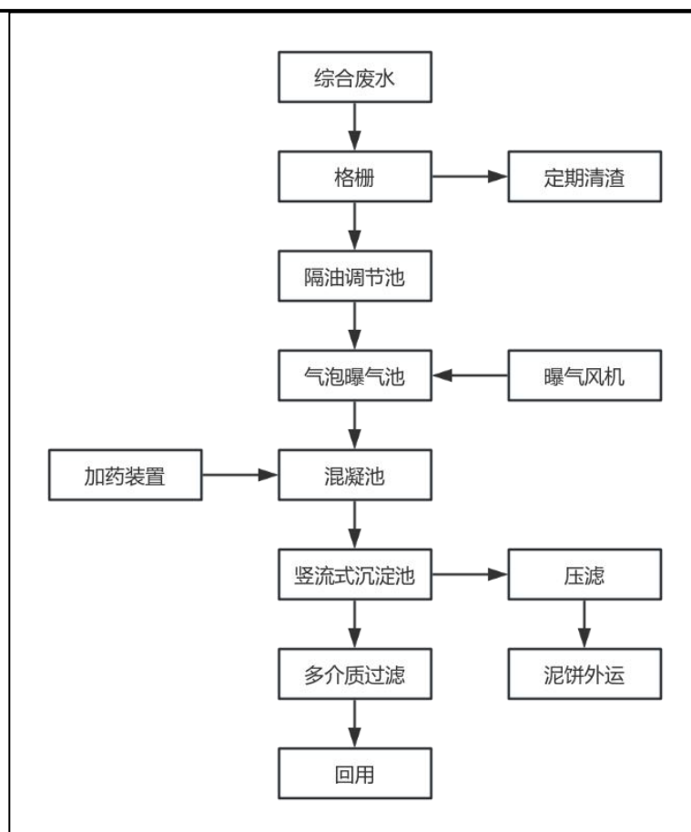
图 4-1 自建污水处理设施工艺流程图
