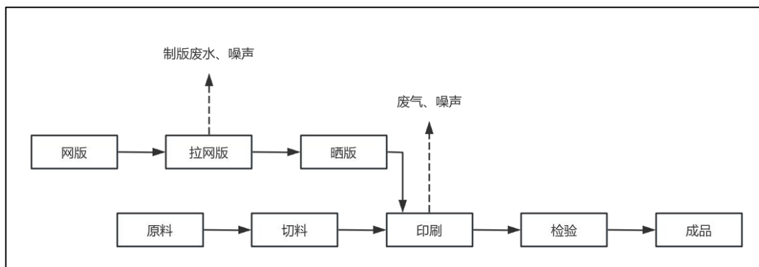
图 2-2 生产工艺流程图
