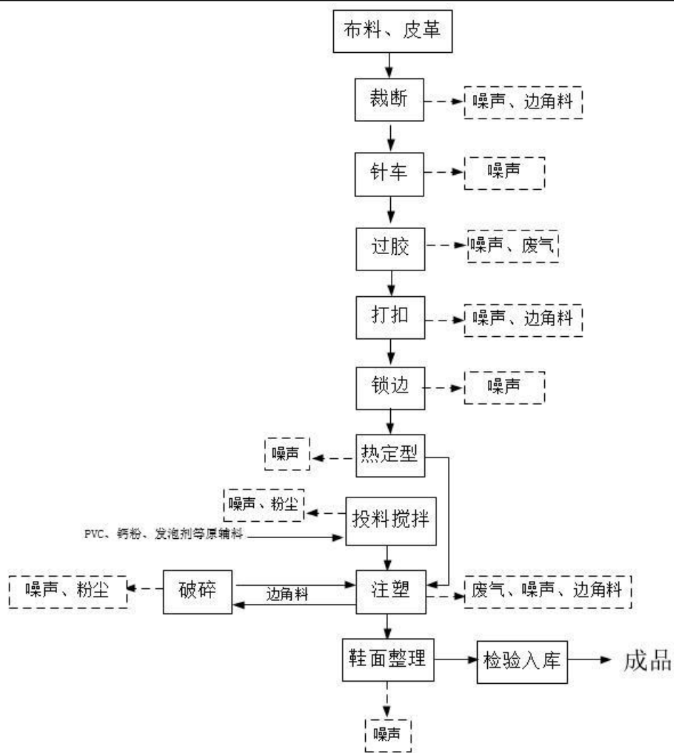
图 2-3 注塑鞋生产工艺
