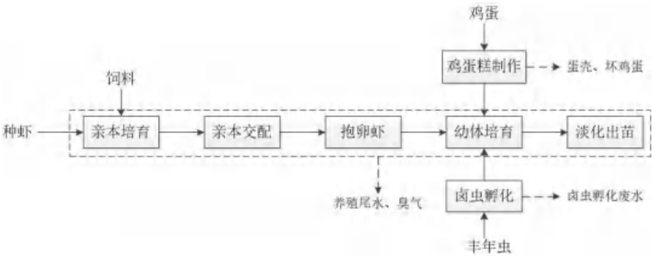
图 2-6 罗氏沼虾育苗工艺流程图
