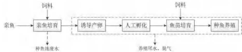
图 2-7 溪鱼育苗工艺流程图
