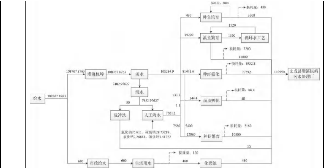
图 2-3 全厂水平衡图 单位：t/a
